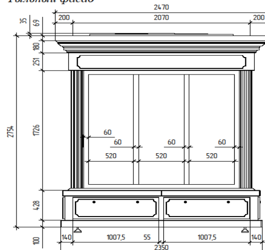
Тыльный фасад
