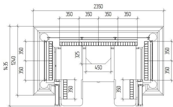
План
