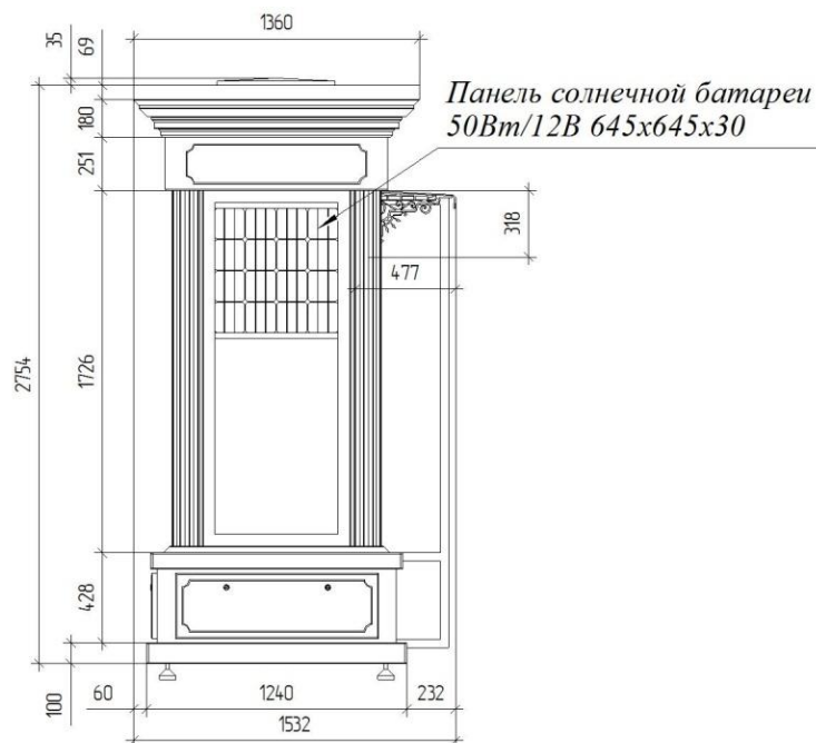
Тыльный фасад
