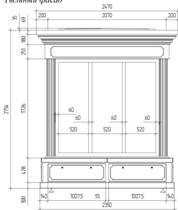
Тыльный фасад
