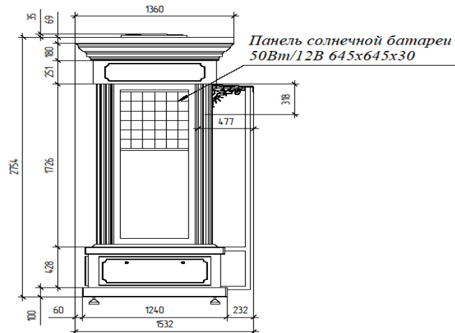
Тыльный фасад
