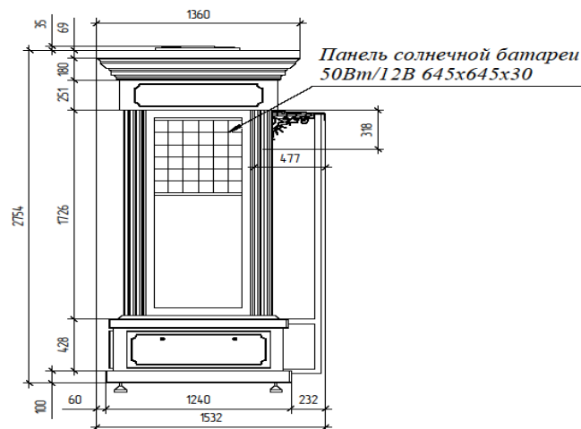
Тыльный фасад
